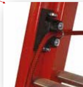
TAQUET COINCEUR ET CORDE Ø 10.5
